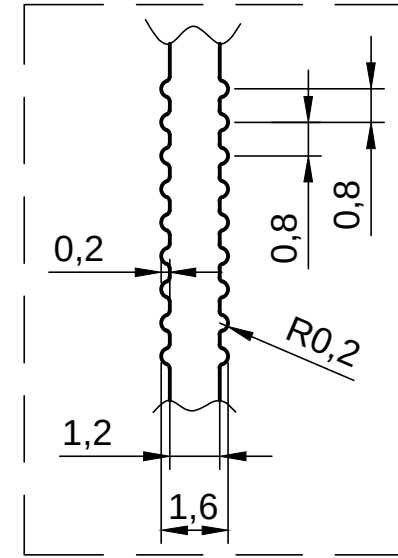
DETAY: A ÖLÇEK: 4/1
