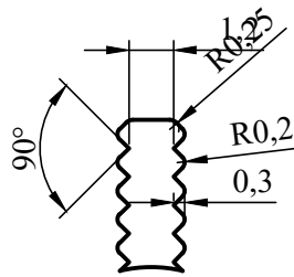
ÖLÇEK 5/1 A/A DETAY
