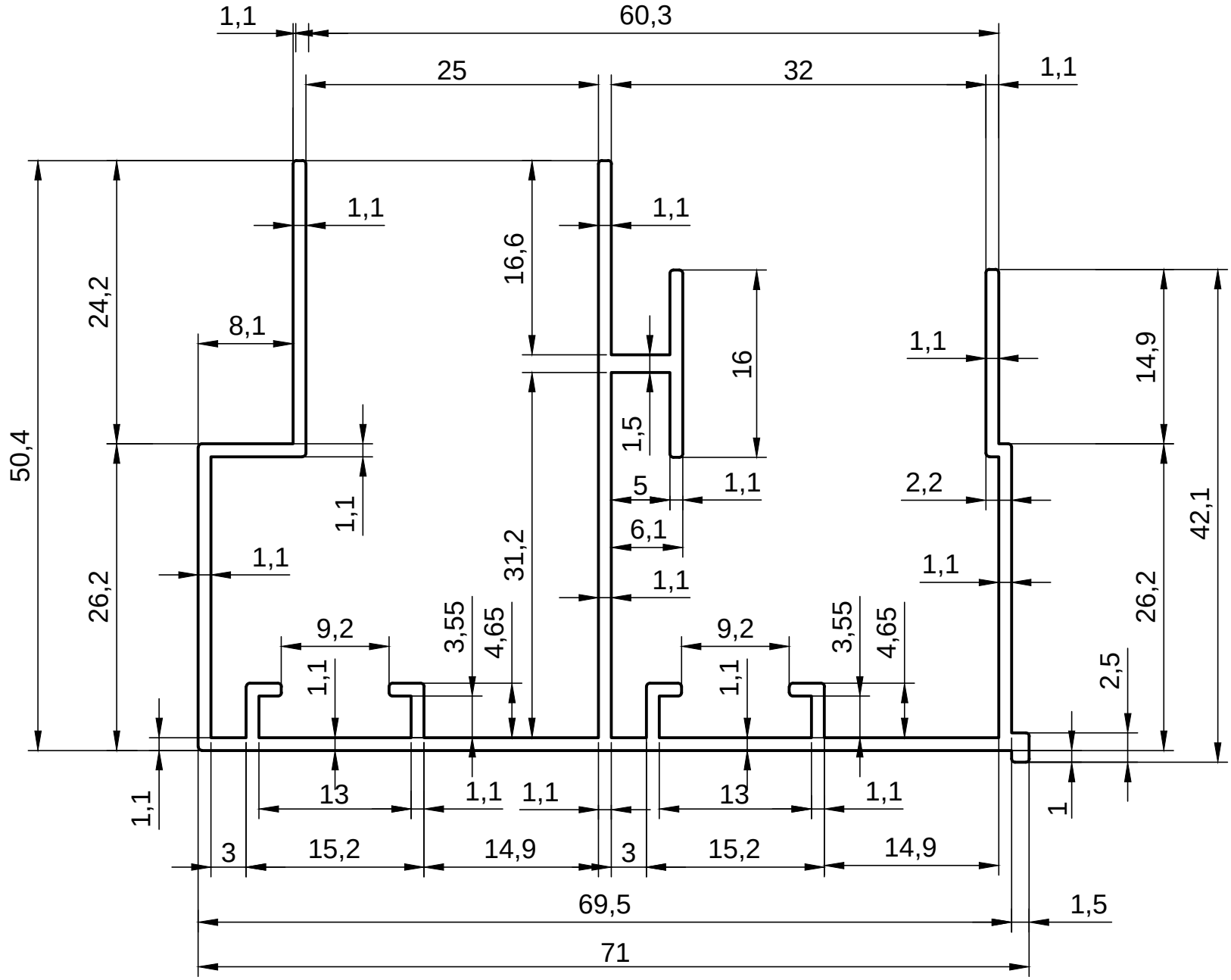
ÖLÇEK 1/1
